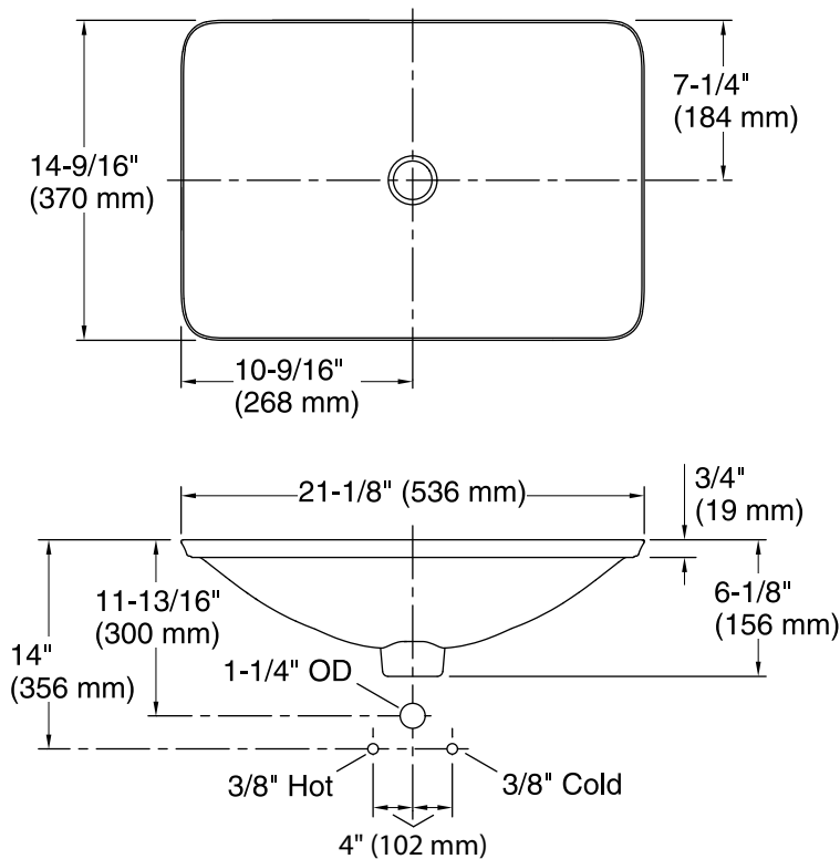
Instalación estándar
